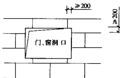
图 6.1.9 (b) 门窗洞口 EPS 板排列
