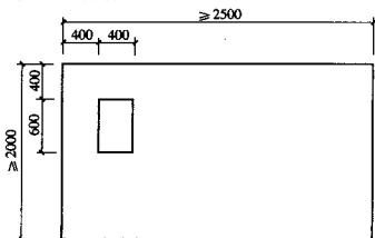
图 A.2.1 试样
