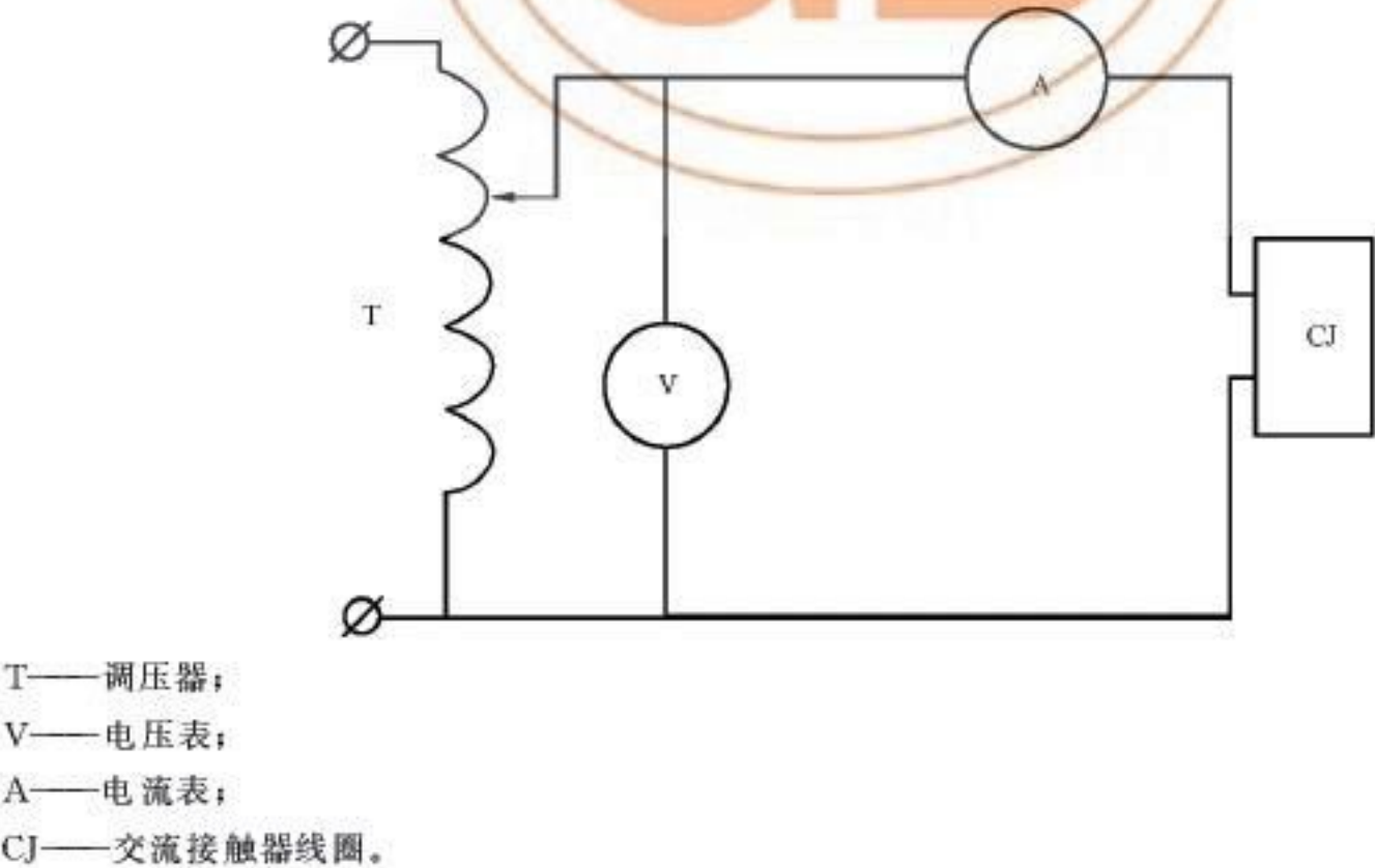
图 1 试验接线图
